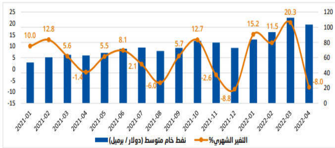
الشكل رقم (05): أسعار النفط الخام
