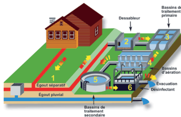
Figure 12: Traitement des eaux usées source: opérateur de traitement des eaux
