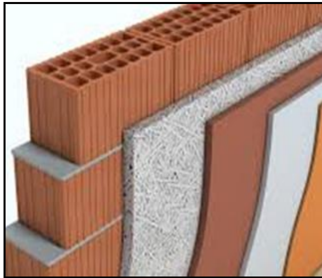
Figure17: Maçonnerie en brique en terre cuite avec isolation en ouate de cellulose
