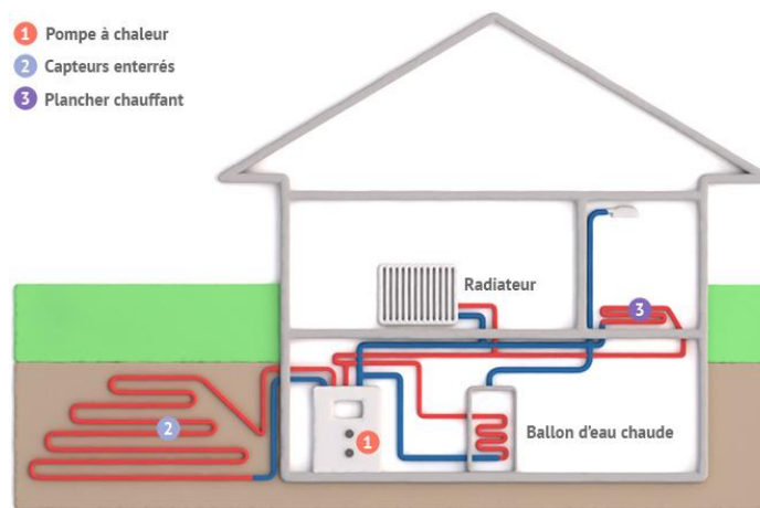
Figure 14: Pompe à chaleur Source: l'iconologie à la maison
