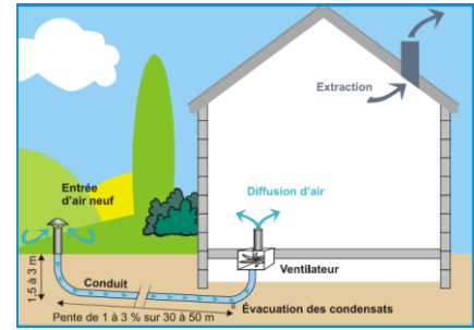
Figure16: Puits canadien source: Domotique puits canadien
