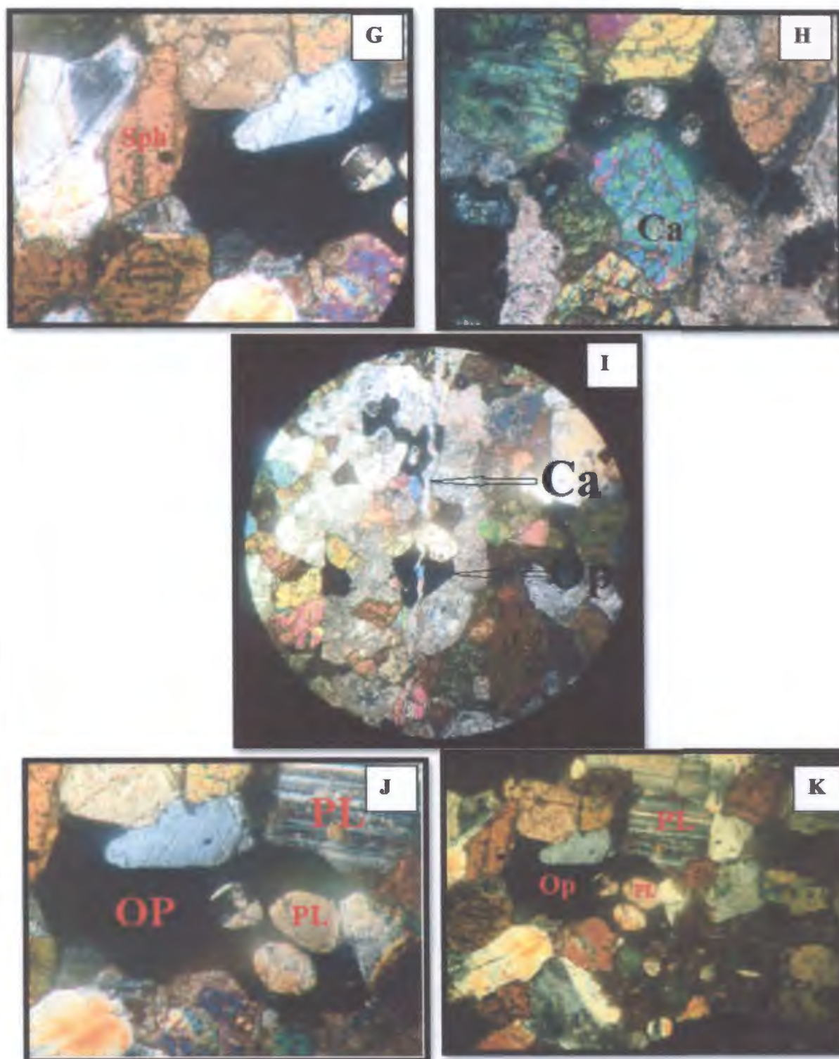
Fig. III.3: Aspect microscopique de Gabbro de Djebel Sendouah.
