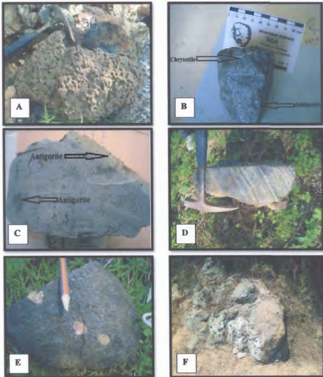
Fig. II.10 : les roche magmatique de complexe volcano-sédimentaire de Djebel Sendouah.
