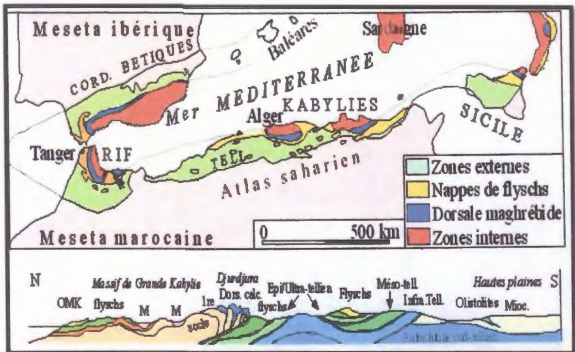
Fig. I.4 : Schéma structural de la méditerranée occidentale. (M. Durand Delga, 1969)
