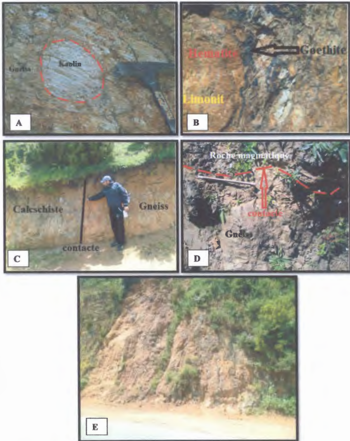
Fig. II.5 : les formations d'Unité du socle de Djebel Sendouah. A) : Kaolin dans les gneiss. B) : minéralisation du socle du Sendouah. C et D) : contact socle- complexe volcano-sédimentaire. E) : Gneiss de Djebel Sendouah.
