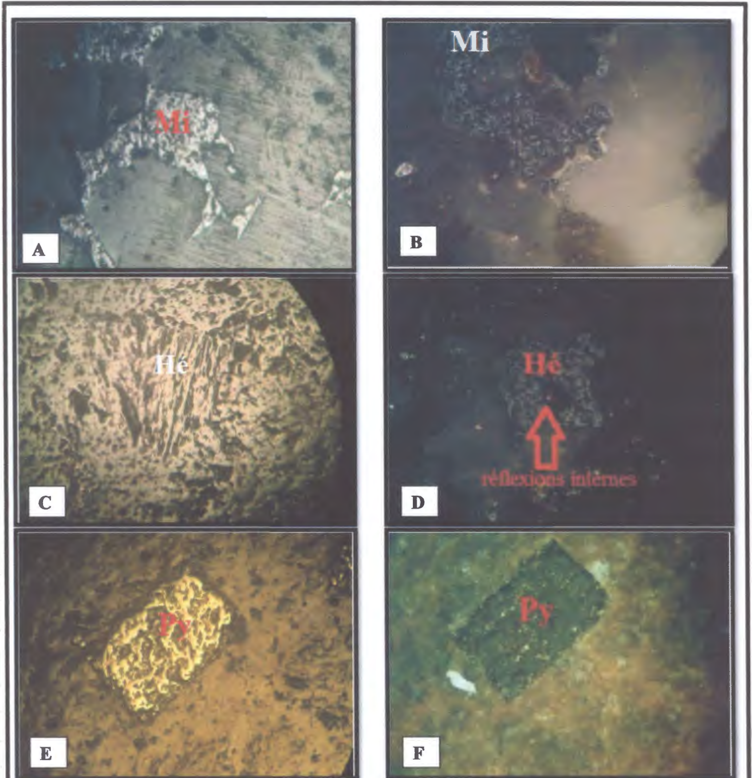
Fig. IV.1 : aspect microscopique de minéralisation de Djebel Sendouah . A, B): Mispickel. C, D): Hématite. E, F): cristaux de Pyrite. Photos section polies (A, C et E : LN. G x 20 ; B, D et F : LP. G x 20)
