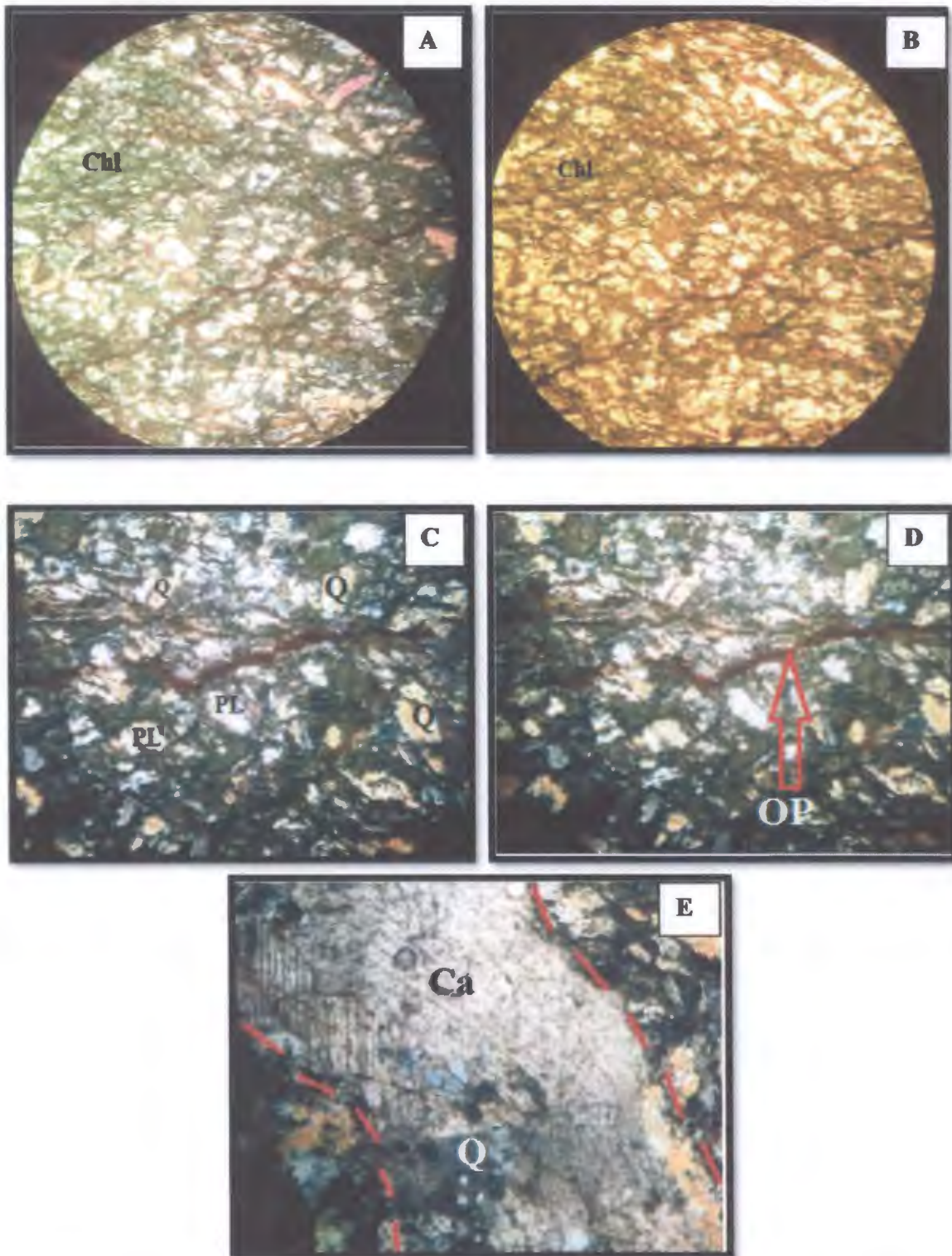
Fig. III.7: Aspect microscopique de Dolérite de Djebel Sendouah.
