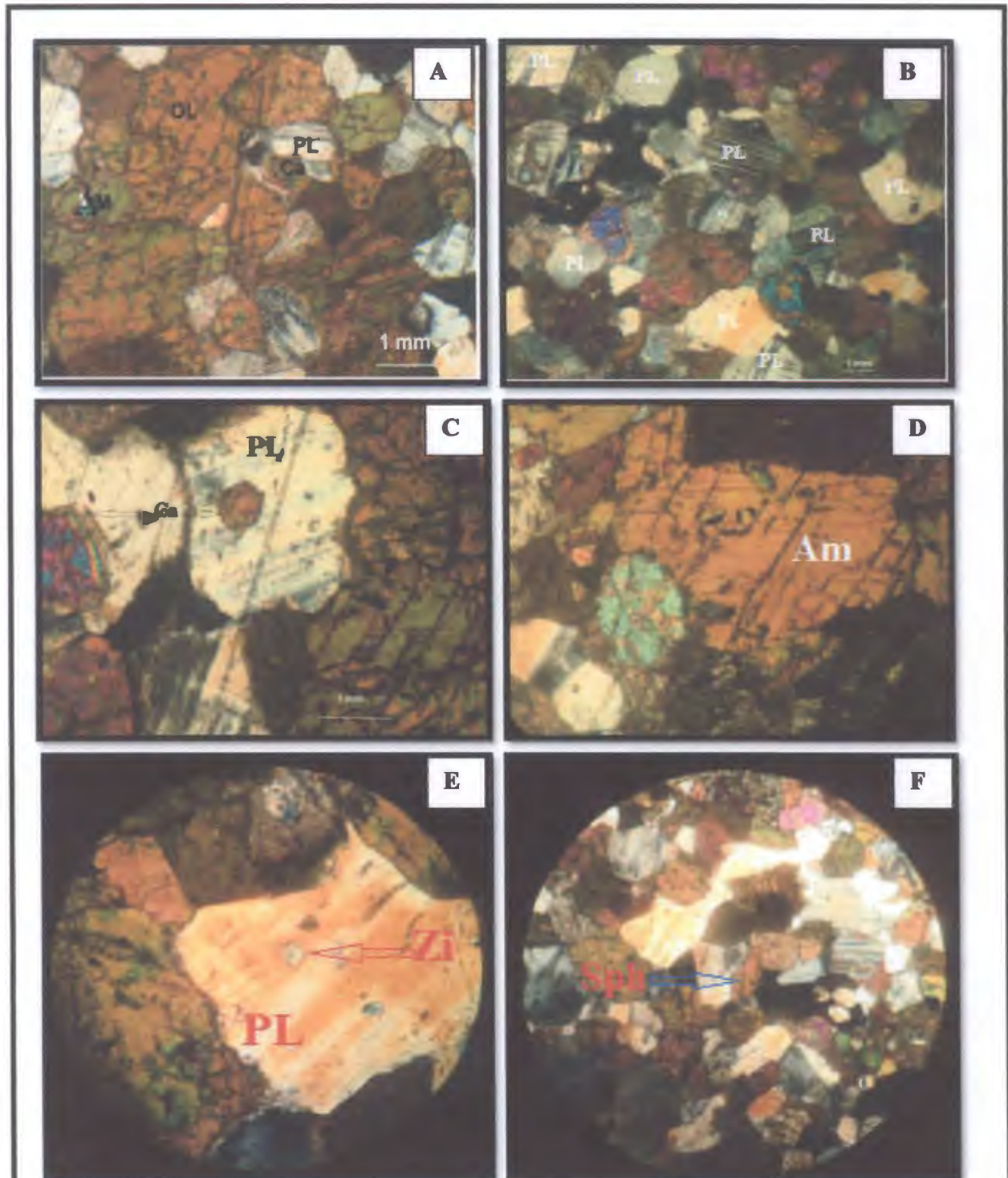
Fig. III.3: Aspect microscopique de Gabbro de Djebel Sendouah.
