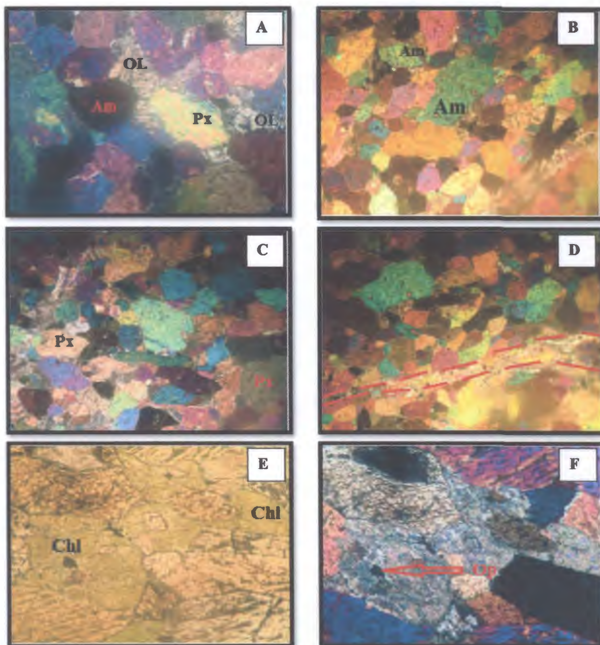
Fig. III.2: Aspect microscopique de Pyroxénolite de Djebel Sendouah.
