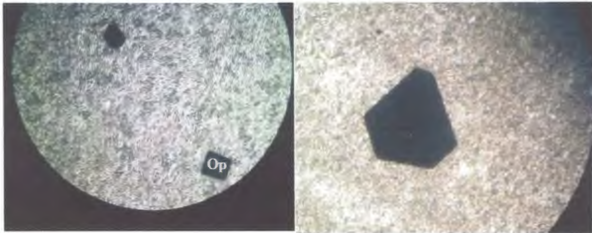
Fig. III.6: Minéralisation dans des Basaltes de texture microlitique (LP. G x5 et 10)
