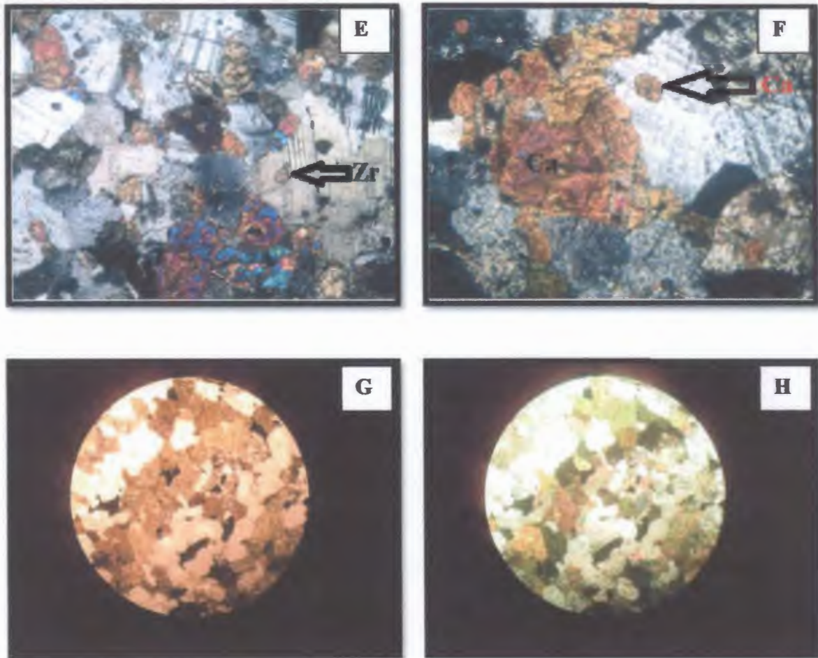
Fig. III.4: Aspect microscopique de Gabbro-lité de Djebel Sendouah.
